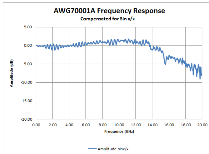
50 GS/s 下的 AWG70001A 频响，从实测数据中以数学方式去掉 Sin x/x 响应
