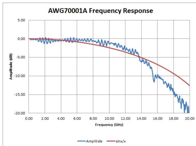
50 GS/s 下的 AWG70001A 测得频响及理想的 Sin x/x 响应
