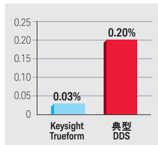
总谐波失真
