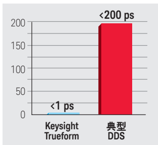
抖动
