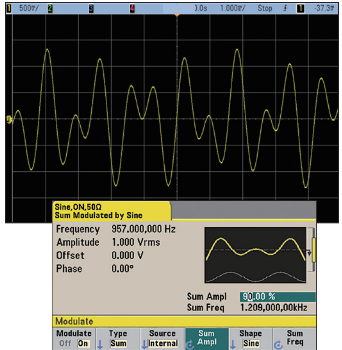
使用调制类型“Sum”进行波形叠加, 从而生成双音信号。
