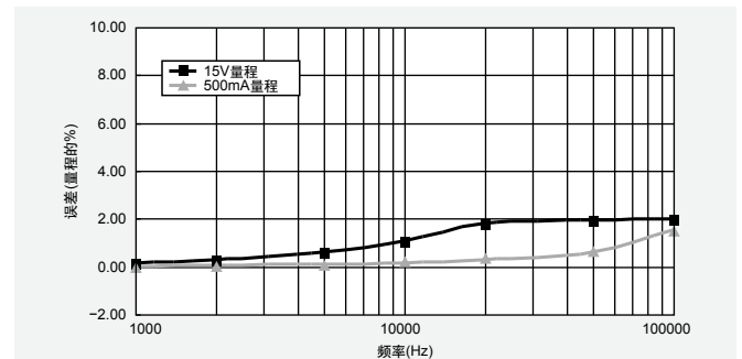
共模电压对读值的影响
